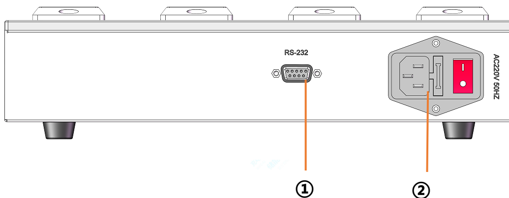
图 2.3.2 ASD652功率计后面板
