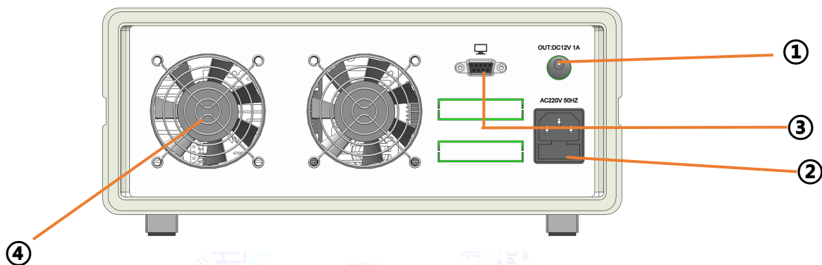
图 2.3.1 909B主机后面板
